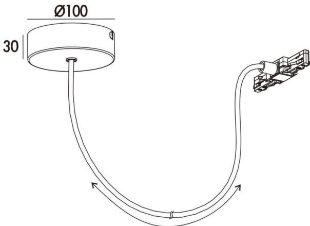
CABLE 2500
